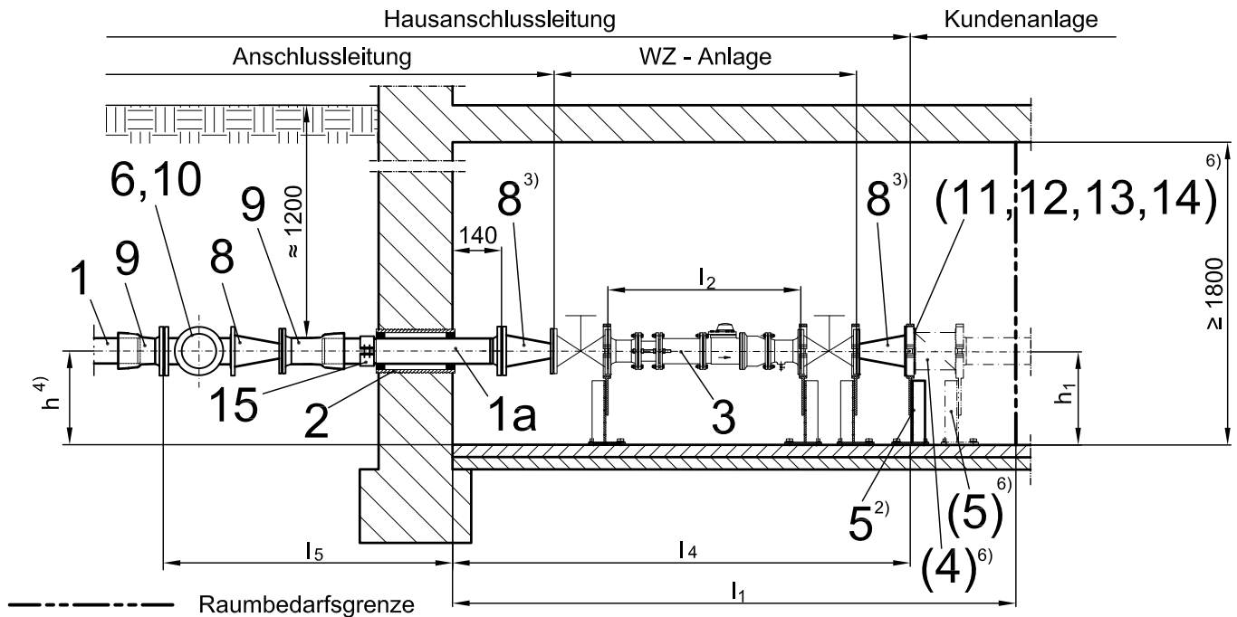
Bild 3 – Fluchtende Bauweise, Anschlussleitungen DN 100, 150, 200, 300 oder 400 Einbau einer Parallel-Groß-WZ-Anlage nach WN 288 oder WN 289 (Bsp. für Parallel-Groß-WZ-Anlage DN 150 nach WN 289 in Anschlussleitung DN 400 dargestellt) (Prinzipskizze)
