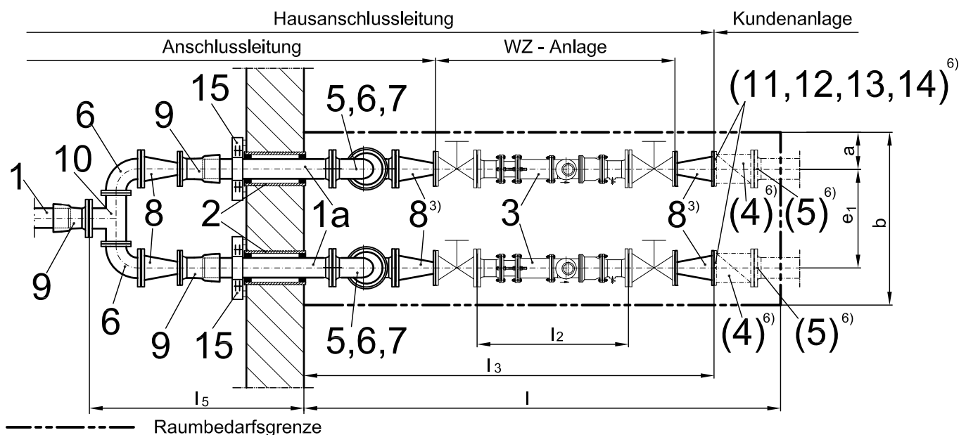
Bild 2 – Grundriss, Anschlussleitung DN 100, 150, 200, 300 oder 400 (Etage dargestellt) Einbau einer Parallel-Groß-WZ-Anlage nach WN 288 oder WN 289 (Bsp. für Parallel-Groß-WZ-Anlage DN 150 nach WN 289 in Anschlussleitung DN 400 dargestellt) (Prinzipskizze)
